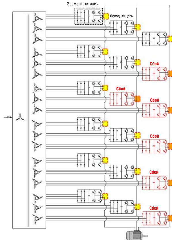
(a) Многоуровневый инвертор в виде H-моста
