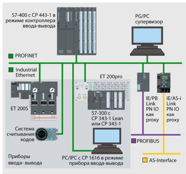
Линейная топология сети PROFINET IO
