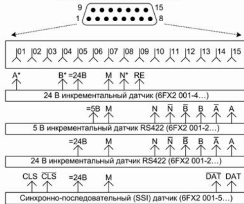
15-полюсные гнезда соединителей CH1, CH2 и CH3
