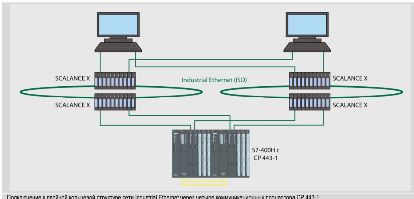
Подключение к двойной кольцевой структуре сети Industrial Ethernet через четыре коммуникационных процессора CP 443-1
