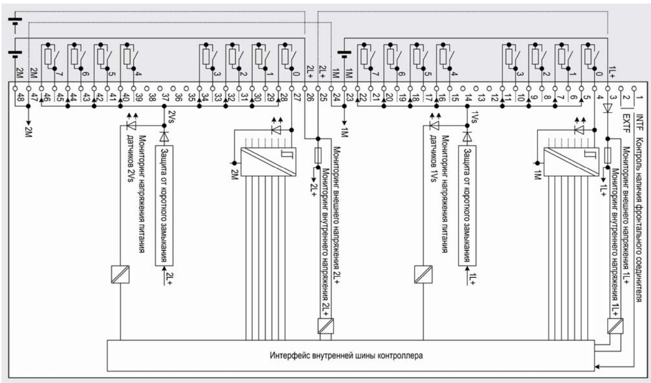
6ES7 421-7BH01-0AB0 (шунтирующее сопротивление датчика 10 ... 18 кОм)
