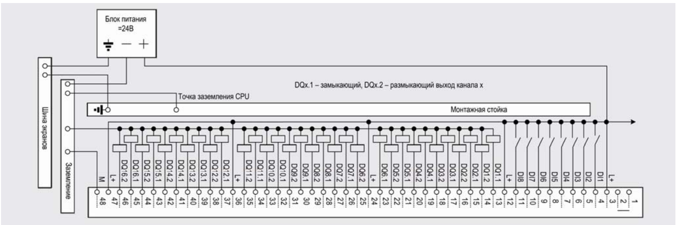
Левый фронтальный соединитель модуля FM 455C
