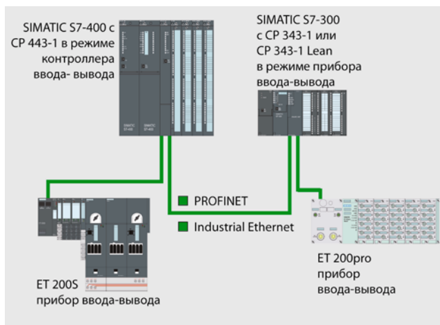
Линейная топология сети PROFINET IO
